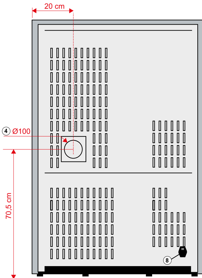
Vista posteriore
