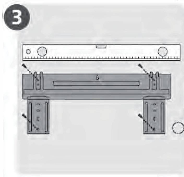
Attaccare la Piastra di Montaggio (Pag. 12)
