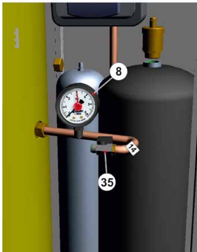
Collegare tubo 14 al rubinetto 3/8" 35 e tubo 13 , inserire manometro 8 .
