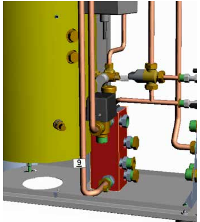
Inserire il compensatore e collegare il tubo 9 (coibentato)
