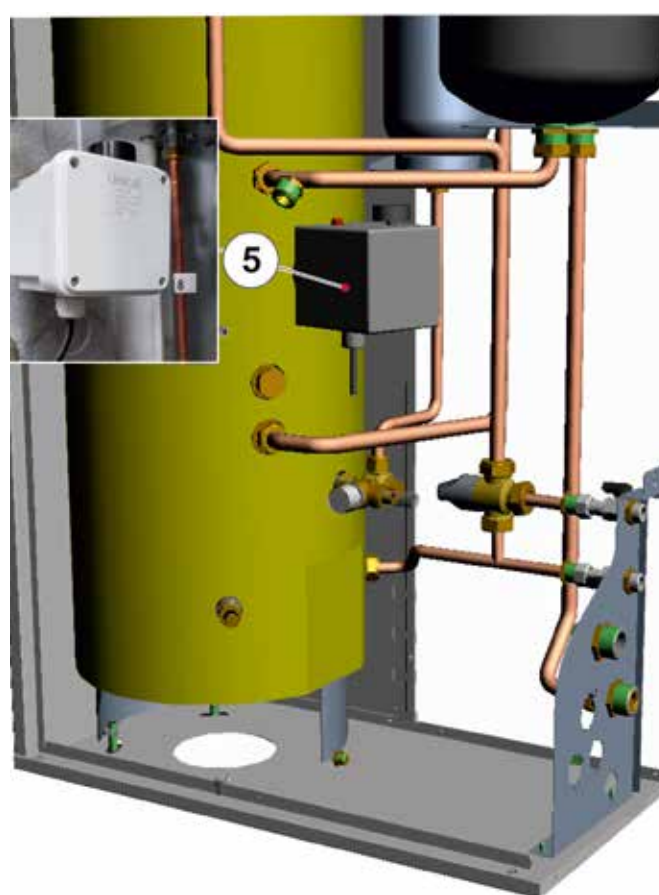
Inserire resistenza di integrazione 5 (Fissare con teflon, canapa, sigillante per raccordi )
