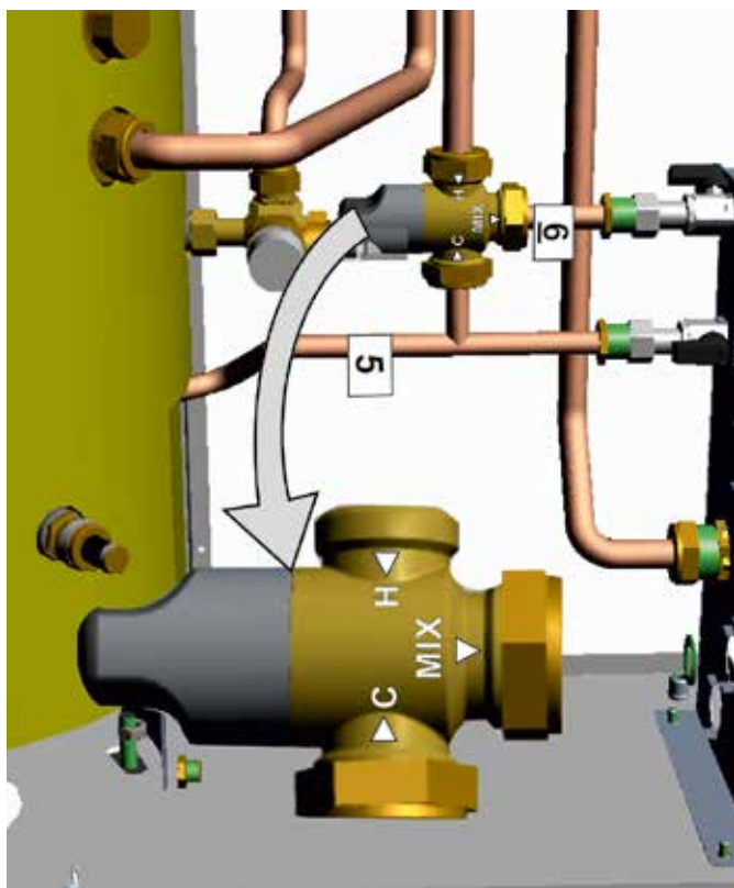
Collegare tubo 6 al rubinetto e alla valvola miscelatrice (attenzione al senso di inserimento) vedi ingrandimento
