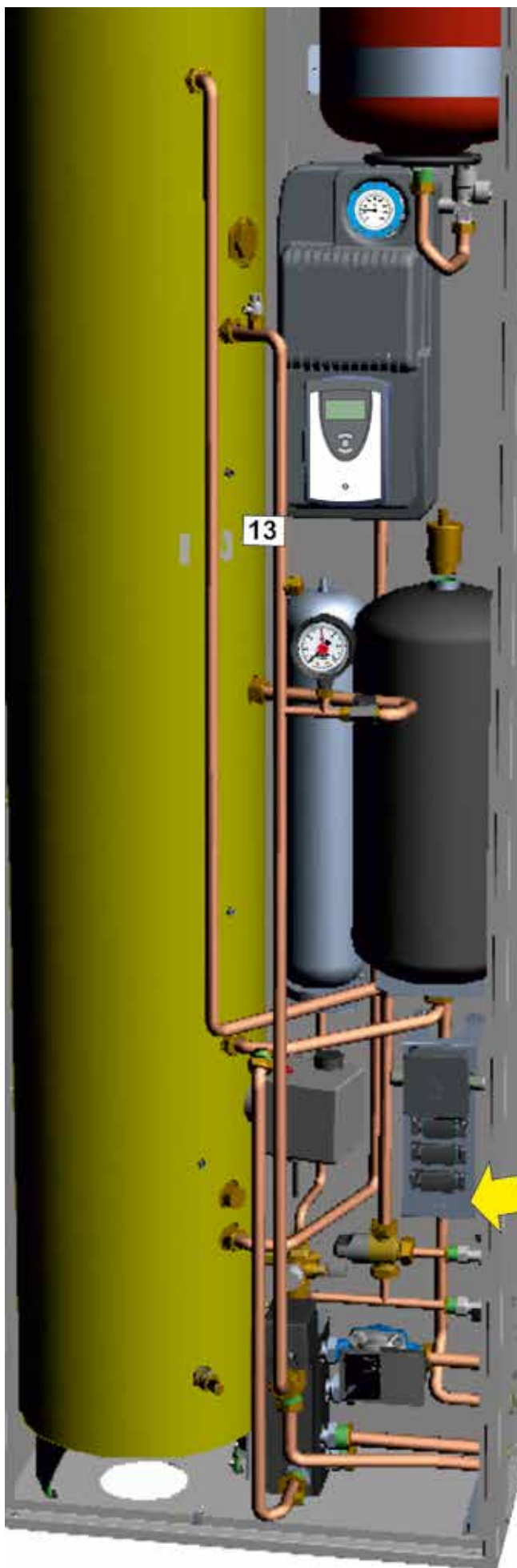
Collegare tubo 13 (coibentato) alla valvola di zona 30
