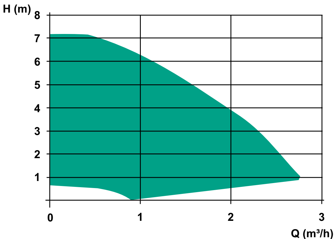
Grafico prevalenza utile impianto al netto delle perdite con Pompa di Calore ON (tubazioni RHP/MHP escluse)
