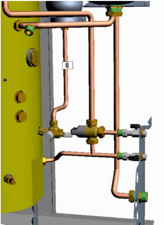
Collegare tubo 8 vaso esp. / valvola sicurezza
