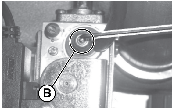
VITE DI REGOLAZIONE POTENZA MINIMA
