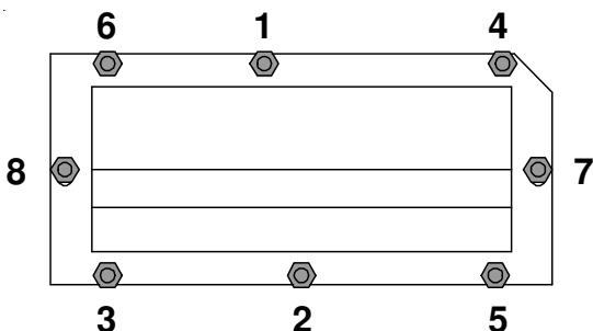
Esempio sequenza di serraggio incrociato per distributore Alkon 28
