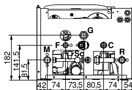
Posizione attacchi ALKON 35S C
