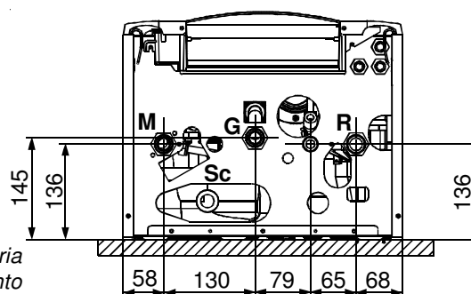
Posizione attacchi ALKON 35S R
