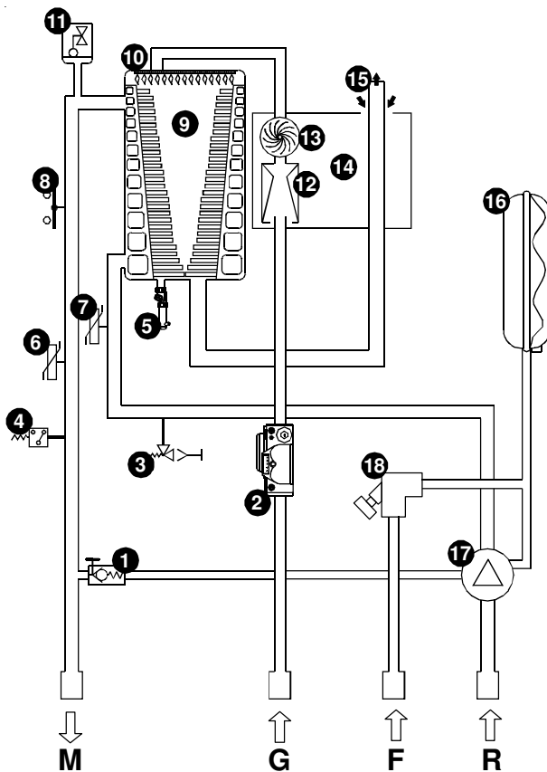
ALKON 35S R
